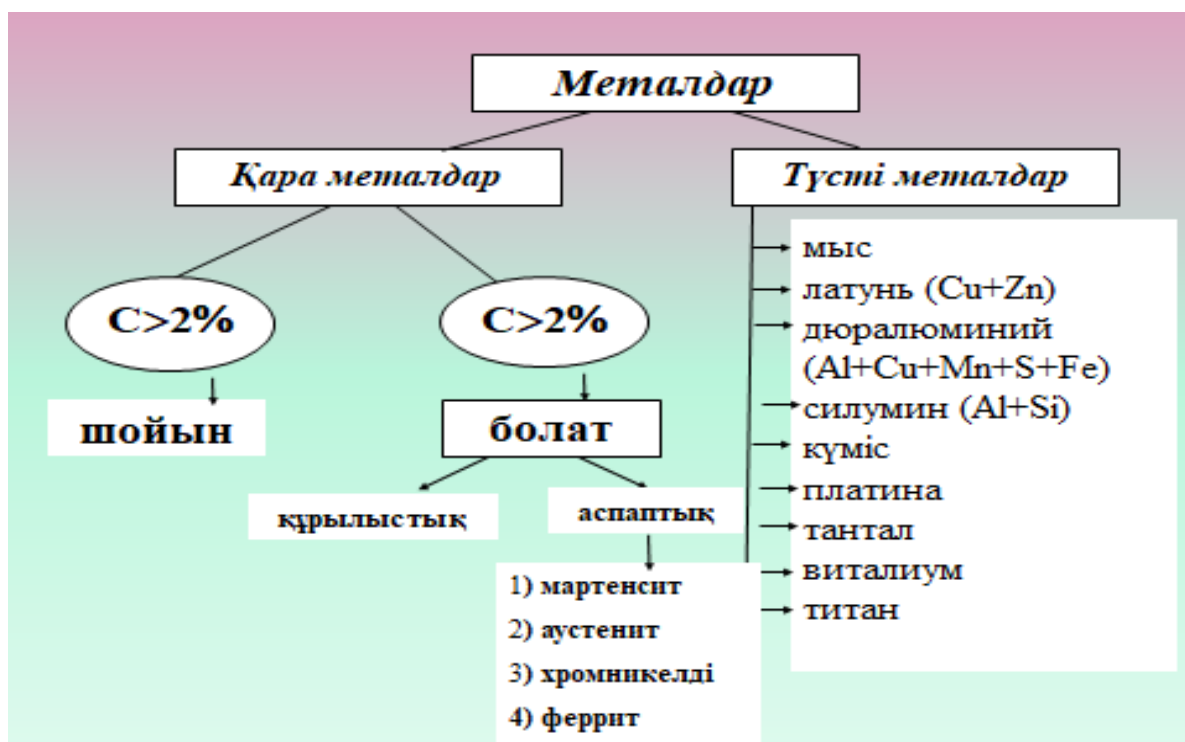
21 сурет-Металлдардың жіктелуі
